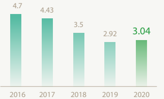
2016-2020 年内蒙古电力集团线损率（ % ）
