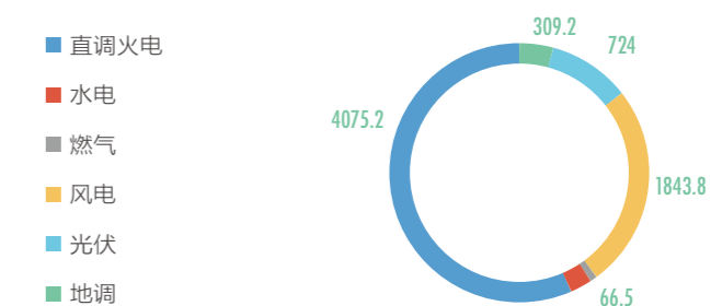
2019年内蒙古电网统调装机容量分布 单位：万千瓦
